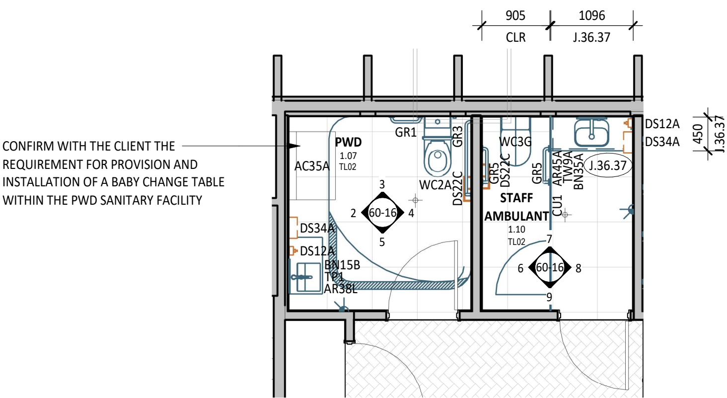
1 PLAN DETAIL 1 : 50
